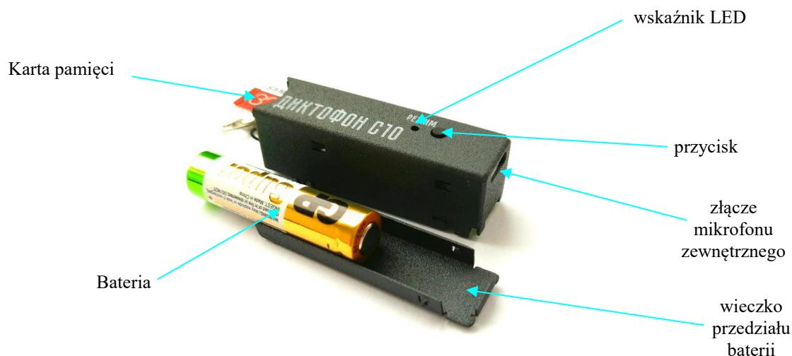
Rys. 2. Rejestrator Soroka-10E
